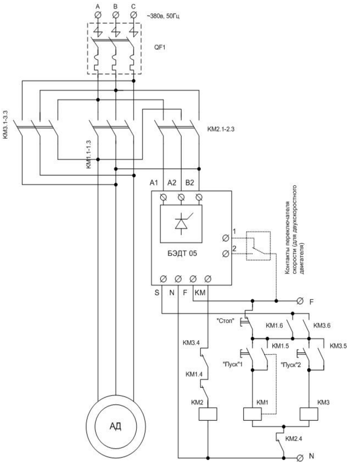
в) типовая схема подключения БЭДТ05 (с реверсом)
