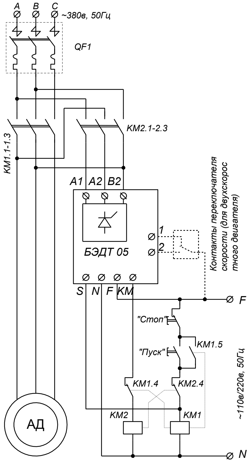
б) типовая схема подключения БЭДТ05
