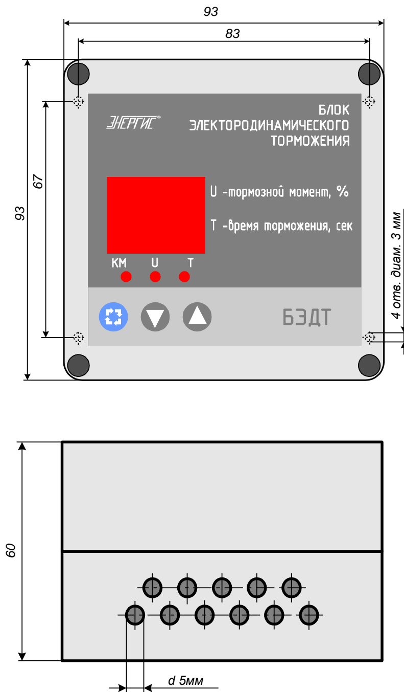
а) внешний вид, габаритные и присоединительные размеры БЗДТ 05-380-32...50-Х
