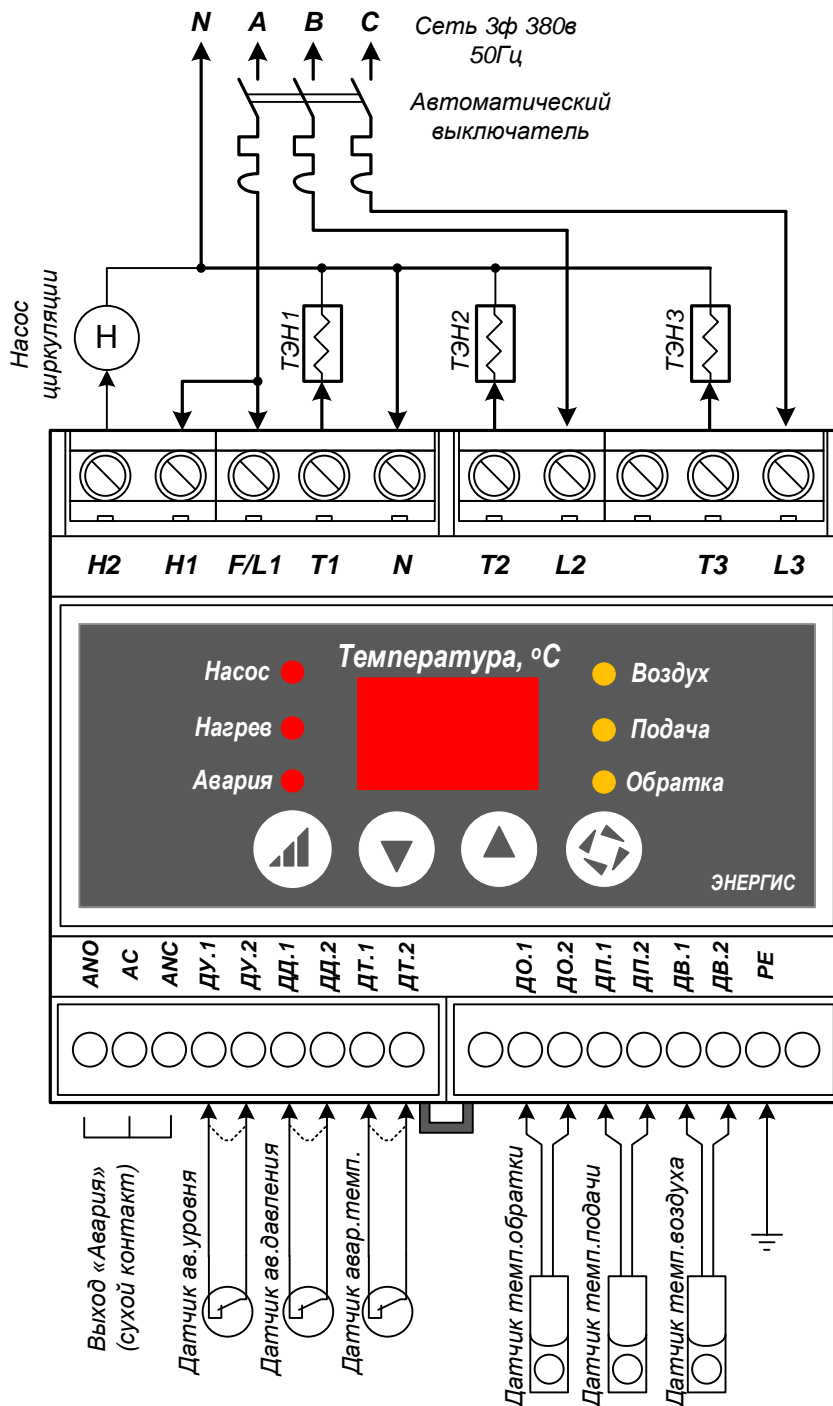
Рисунок 3. Схема подключения
