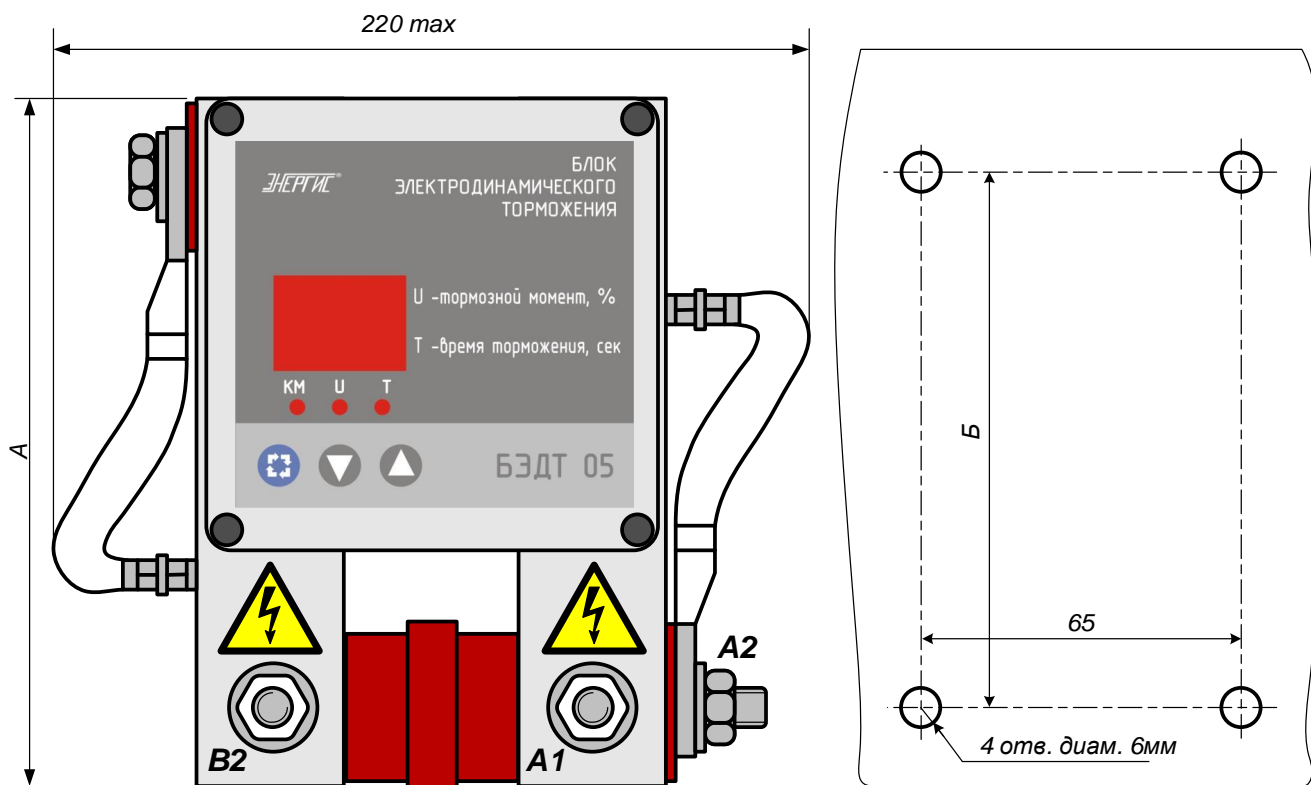
Сверление отверстий для монтажа БЭДТ 05 на монтажную панель
