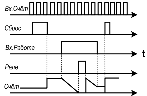
Рисунок 3. СД-1-XX.3. Диаграммы работы.
