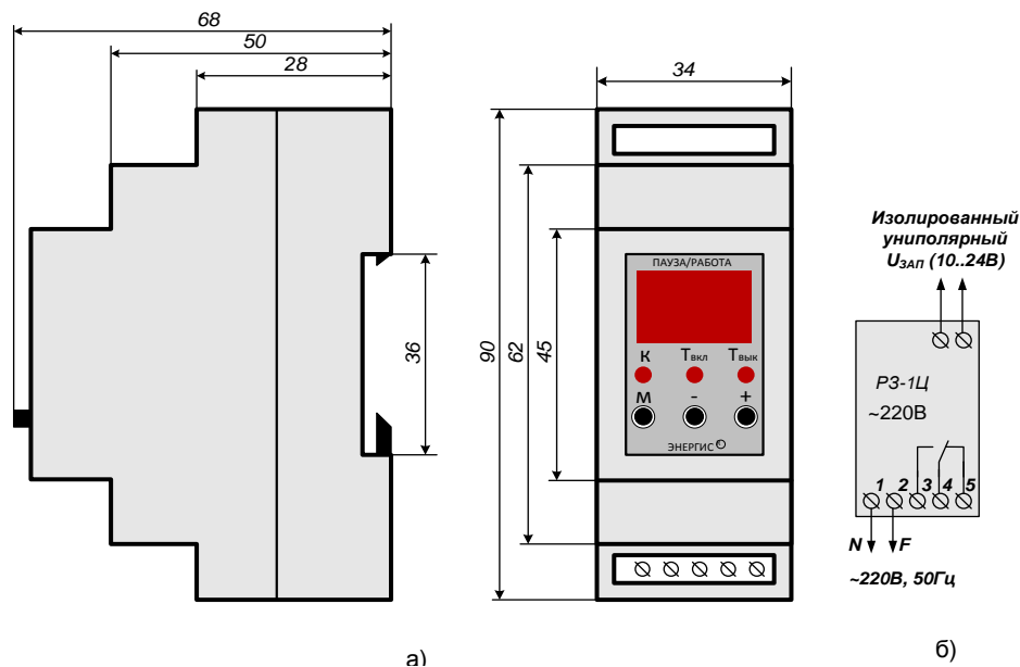
Рисунок 2. РЗ-4Ц. а) габаритные размеры, б) схема подключения РЗ-4Ц.
