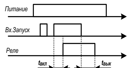
Рисунок 1. РЗ-4. Диаграммы работы.
