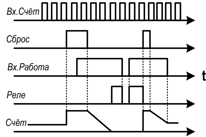
Рисунок 3. СД-1-ХХ.1. Диаграммы работы.
