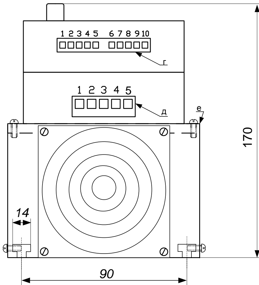
Рисунок 1. ТРН-40-ЦВ. Габаритные и установочные размеры
