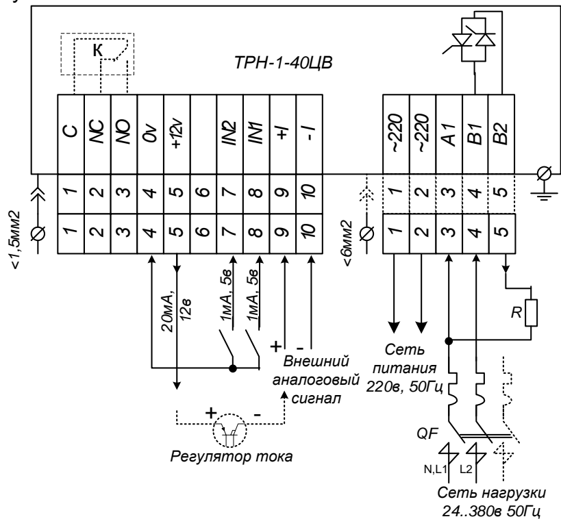
Рисунок 3. Схема подключения.
